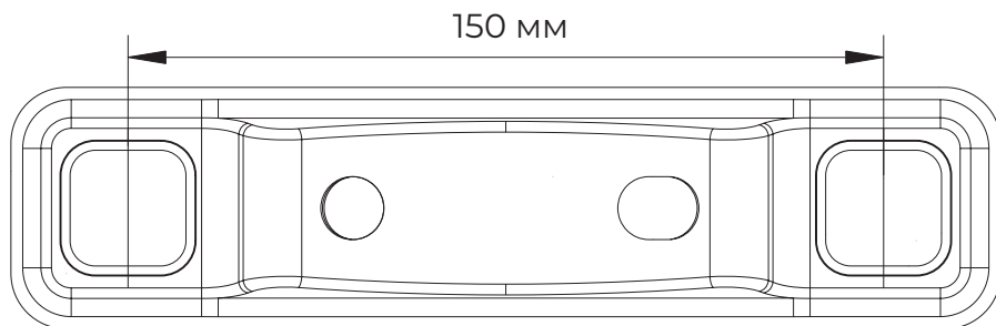
Рис. 6. Кронштейн крепления
